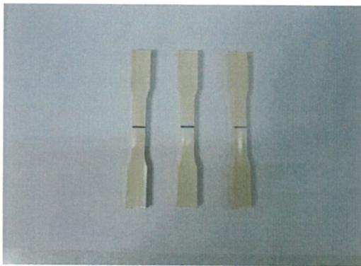
試験片(HIVP50)
