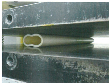
1/2偏平時(HIVP50(ネジ接合))
