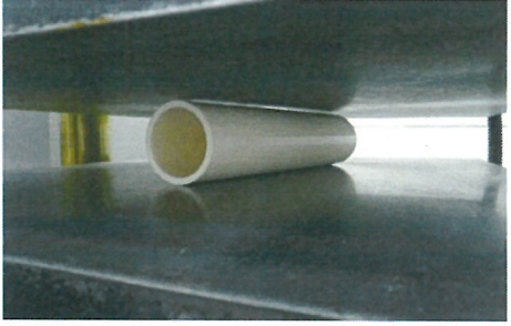
試験状況 (HIVP50スリット入り)
