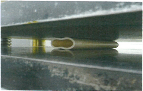
50%偏平時 (HIVP50スリット入り)
