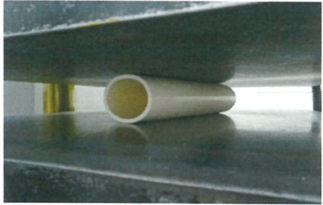
10%偏平時 (HIVP50スリット入り)
